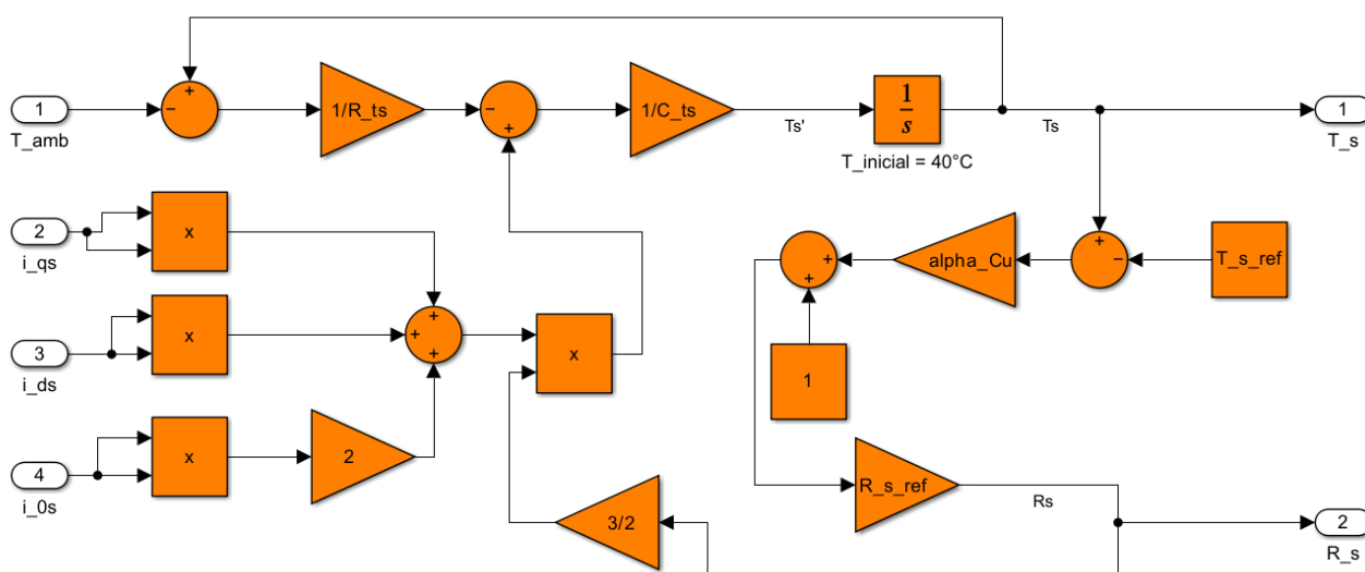
Figura 5: Subsistema térmico
